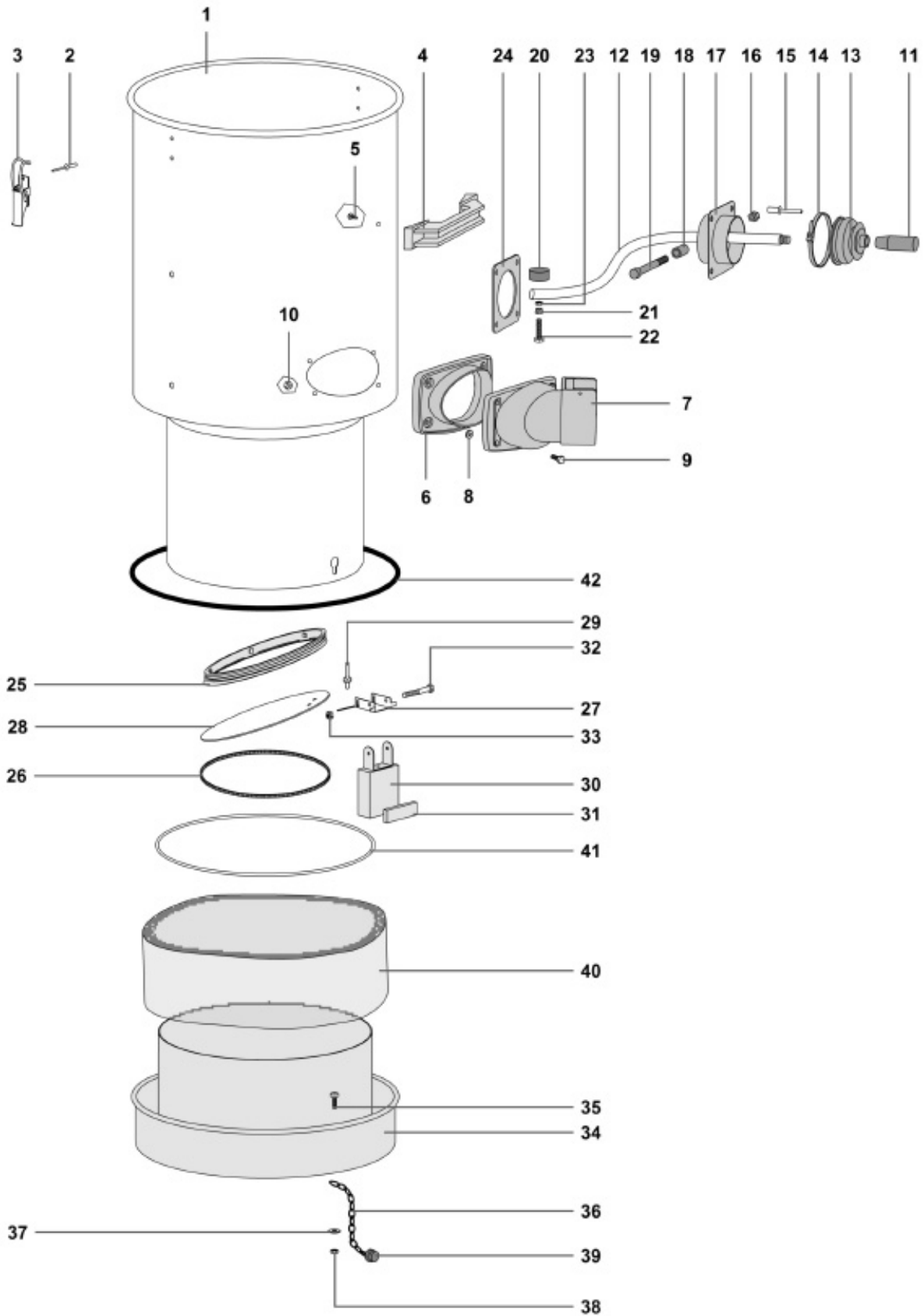
Abb. 30: Ersatzteilzeichnung 5
