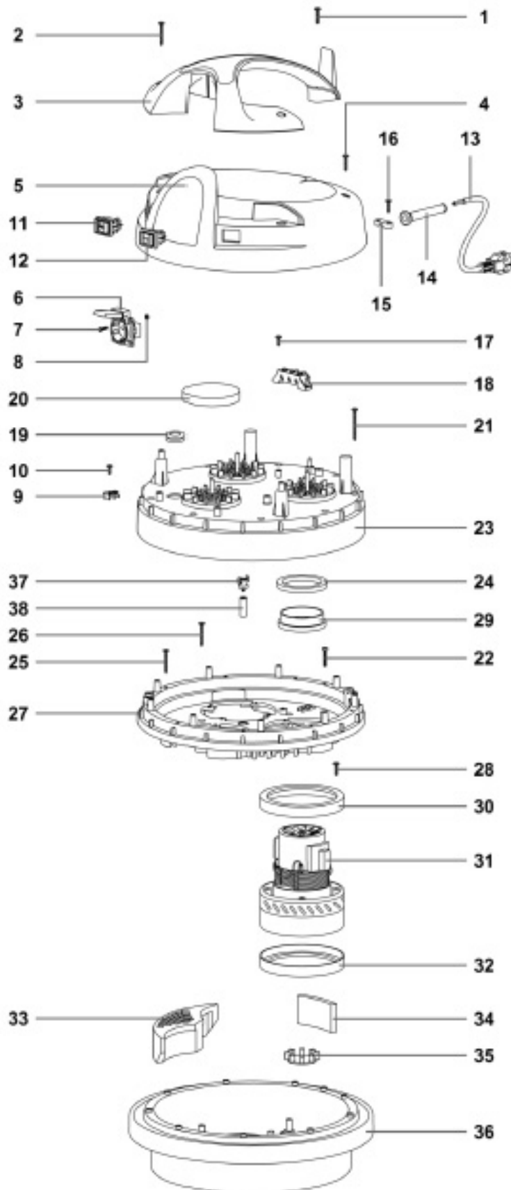
Abb. 28: Ersatzteilzeichnung 1
