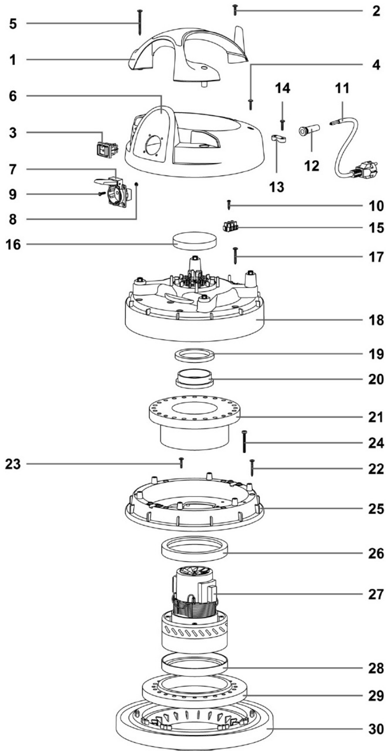
Abb. 22: Ersatzteilzeichnung 1
