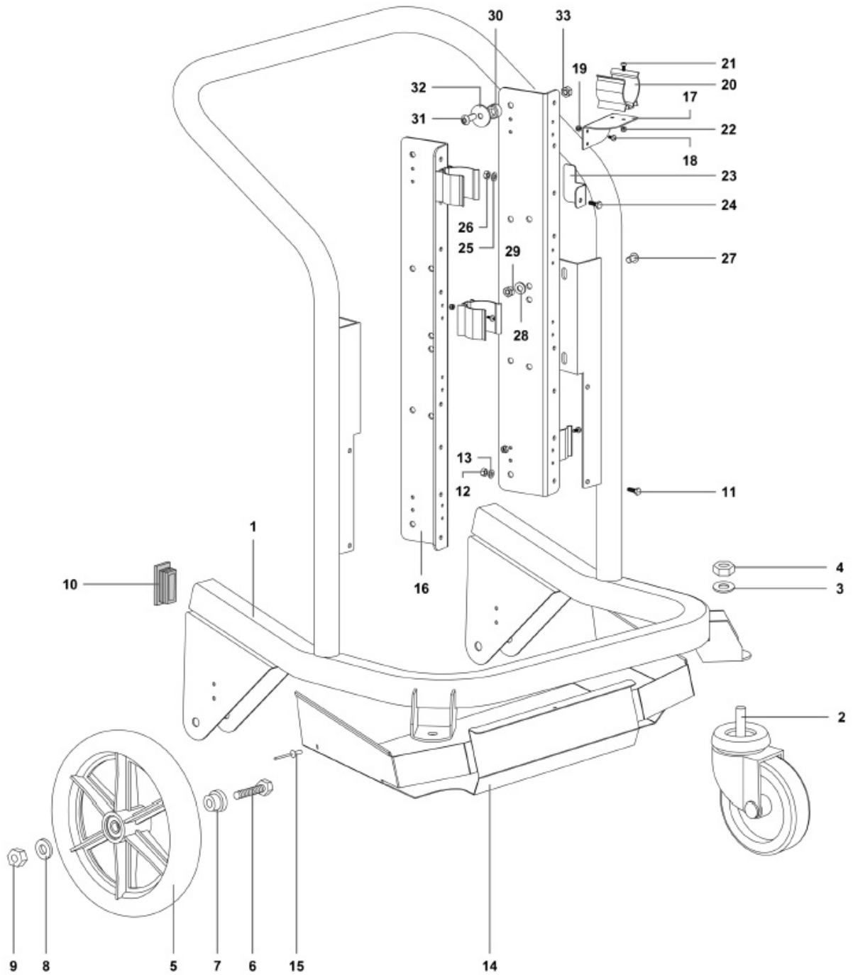
Abb. 31: Ersatzteilzeichnung 6
