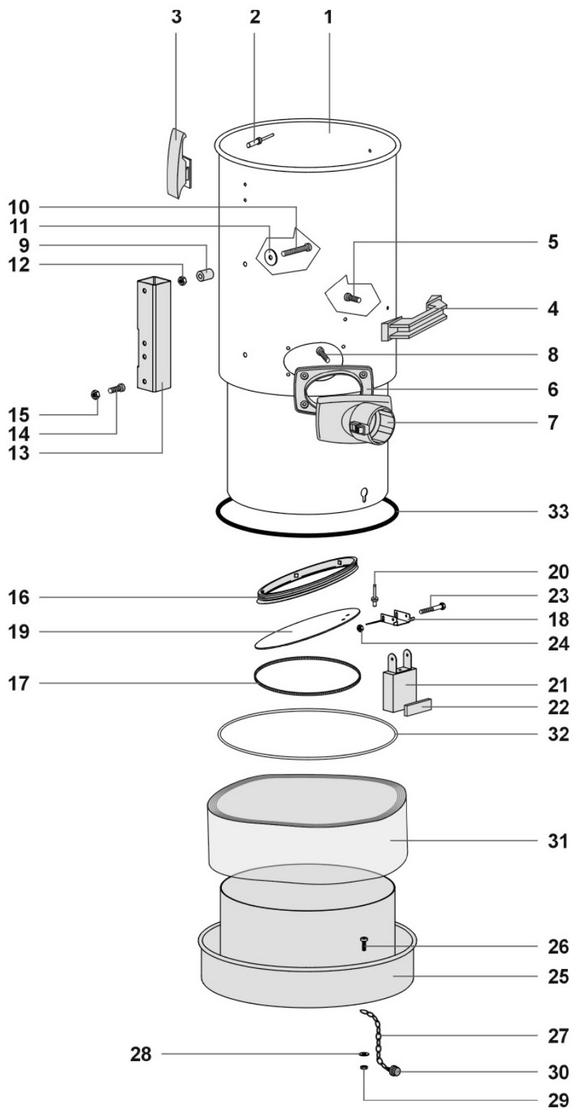
Abb. 23: Ersatzteilzeichnung 2
