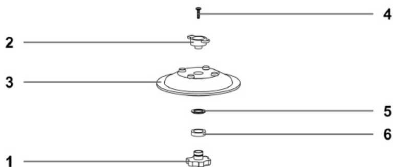
Abb. 29: Ersatzteilzeichnungen 2, 3 und 4
