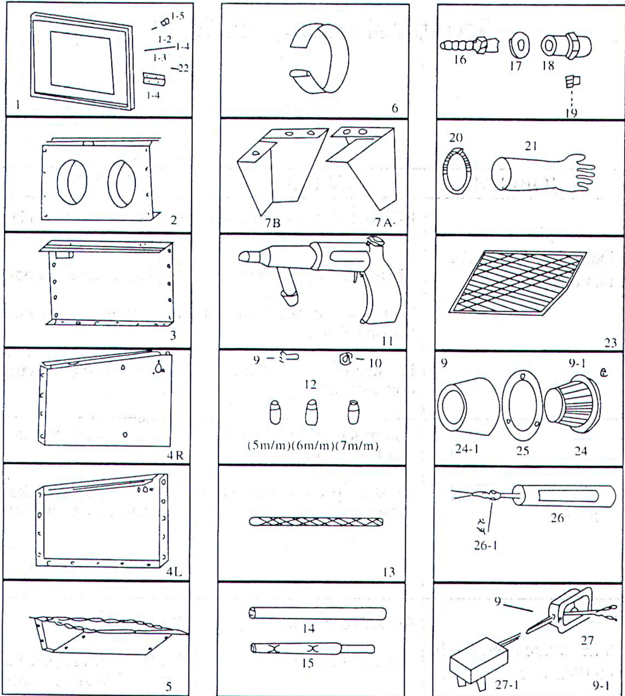
Abb. 13: Ersatzteilzeichnung SSK 1
