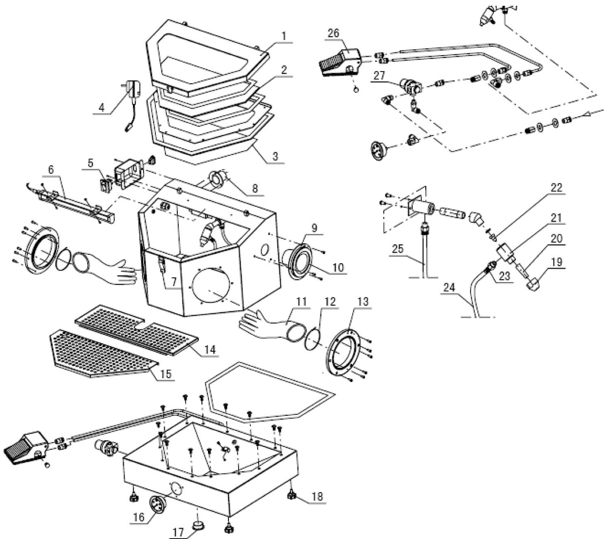
Abb. 14: Ersatzteilzeichnung SSK 1.5
