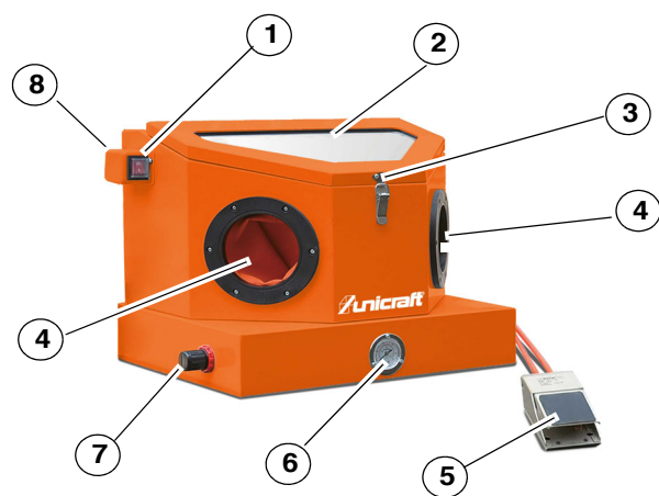
Abb. 4: Sandstrahlkabine SSK 1.5
