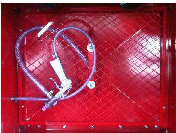
Abb. 8: Ablagegitter
