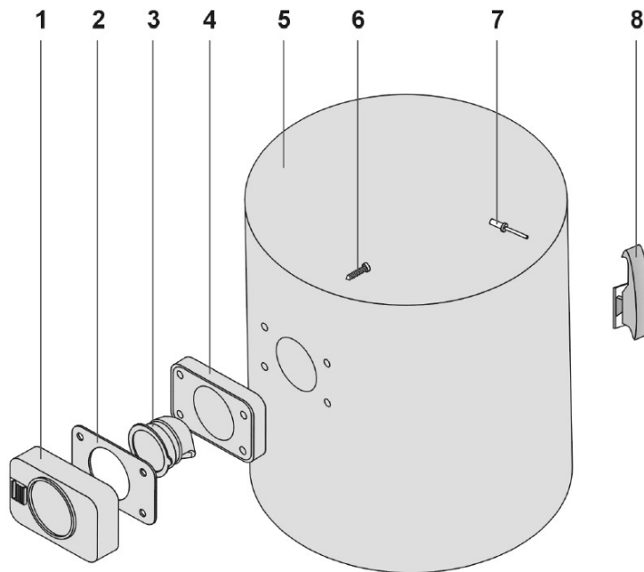
Abb. / Fig. 2: Ersatzteilzeichnungen 2 / Spare parts drawings 2
