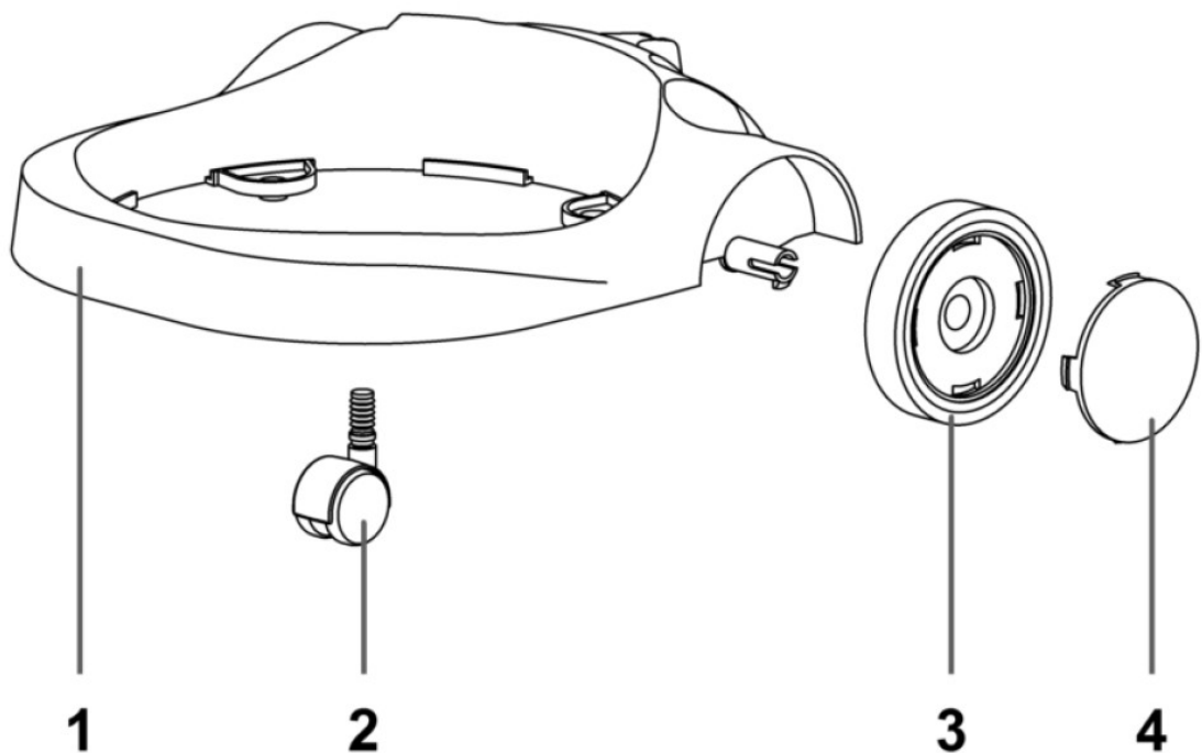
Abb. / Fig. 3: Ersatzteilzeichnungen 3 / Spare parts drawings 3
